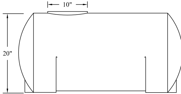
ELEVATION
